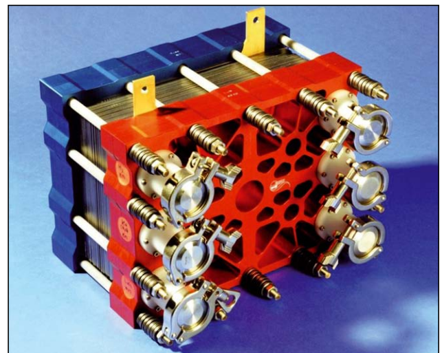
Abb. 5: Vom ZSW entwickelte Brennstoffzelle
