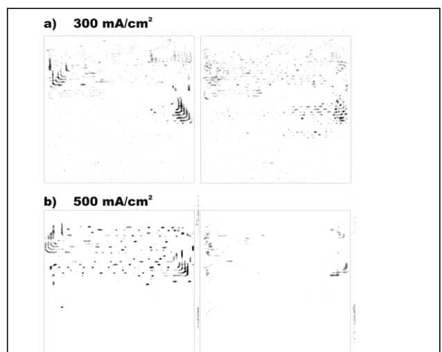
Abb. 10: einzelne Querschnitte durch das Tomogramm eines 3-fachen Brennstoffzellen-Stacks. Die Querschnitte zeigen die Wasserverteilung in einer der Zellen auf der Kathodenseite (jeweils linkes Bild) und der Anodenseite (jeweils rechtes Bild). a) Stromdichte i_0=300 \text{ mA/cm}^2 ; b) bei i_0=500 \text{ mA/cm}^2 . Trotz erhöhter Wasserproduktion aufgrund der höheren Stromdichte ist durch den „electro-osmotic drag“ die Befeuchtung auf der Anodenseite deutlich reduziert.
