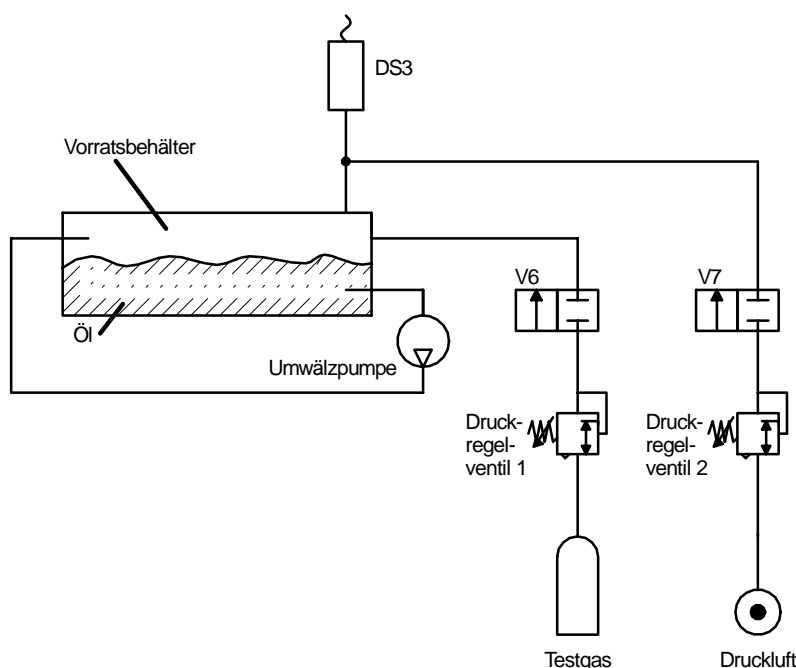
Bild 3: Funktionsprinzip der TLF-Prüfmediumaufbereitung
