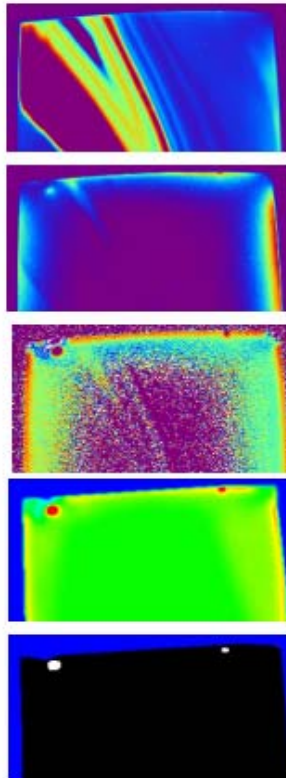
Abbildung 14: Automatisierte Auswertung der Prüfung. Die Risse sind im endgültigen Auswertebild als weisse Puknkte zu erkennen.
