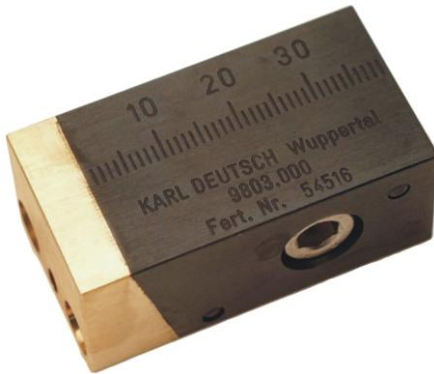
Bild 1: Vergleichskörper 1 (gem. DIN EN ISO 9934-2 [4]) (früher MTU Testkörper)
