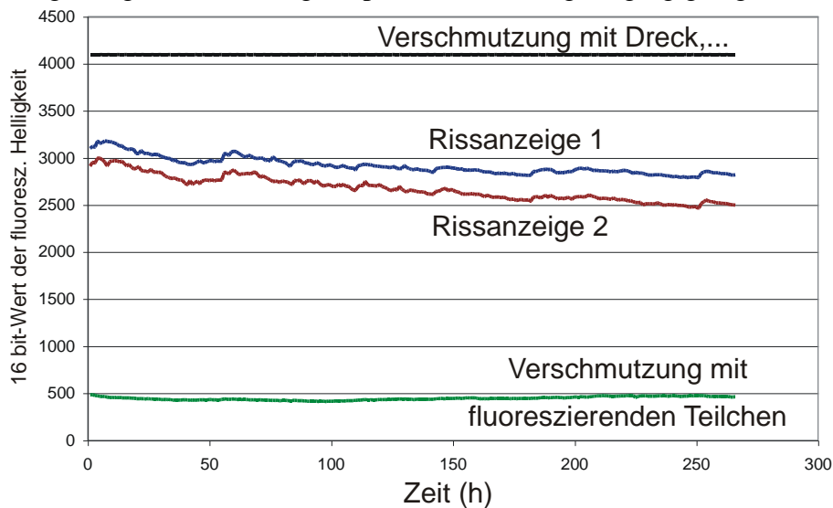
Bild 12: Messergebnis mit sinkender Anzeigeempfindlichkeit.
