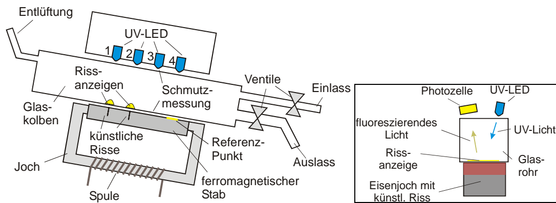
Bild 5: Aufbau der automatischen Überwachung fluoreszierender Prüfmittel.
