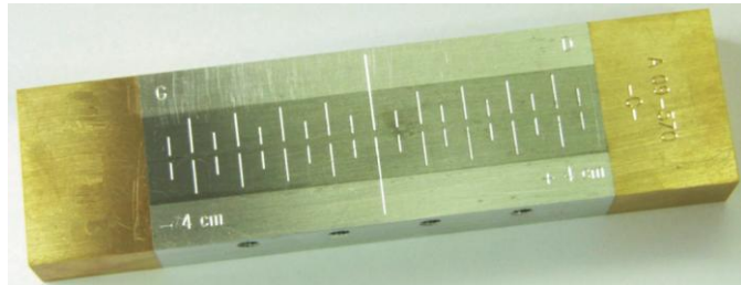
Bild 2: Vergleichskörper 2 (gem. DIN EN ISO 9934-2 [4])
