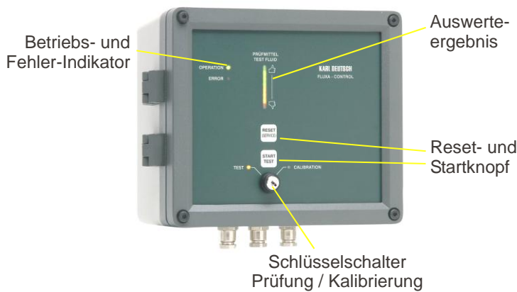
Bild 11: Bedienelemente: FLUXA-CONTROL
