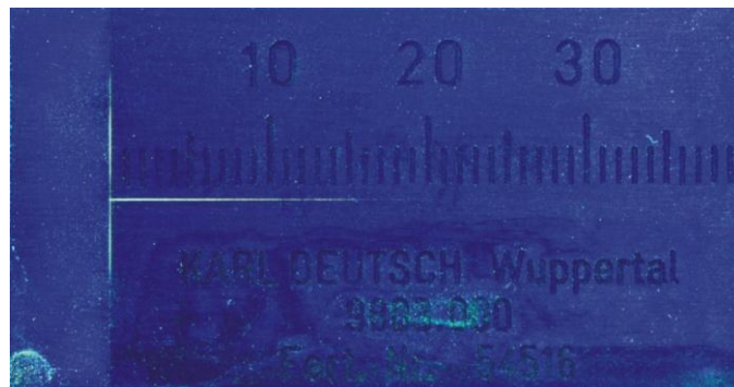
Bild 4: Anzeige am FLUXA-Testkörper unter UV-Licht
