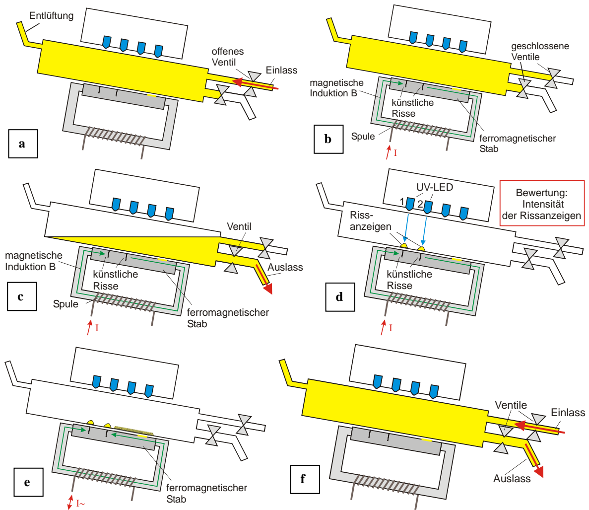
Bild 6: Prinzipieller Ablauf einer Vergleichsmessung mit FLUXA-CONTROL.
