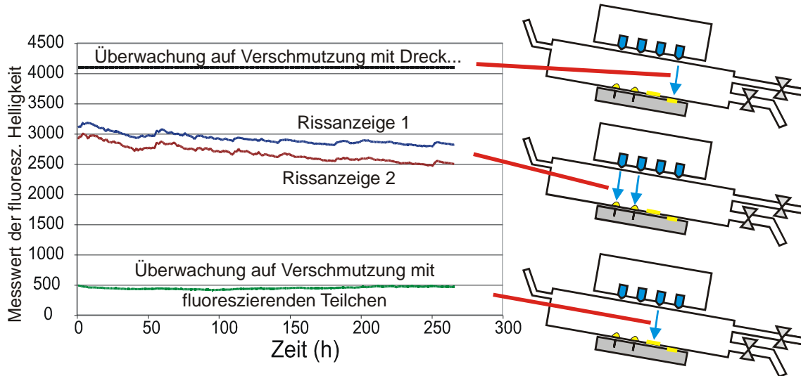
Bild 7: Messwerte in den vier Kanälen (UV-LEDs und Fozozellen).
